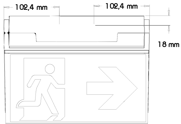
Ansicht Hinten
