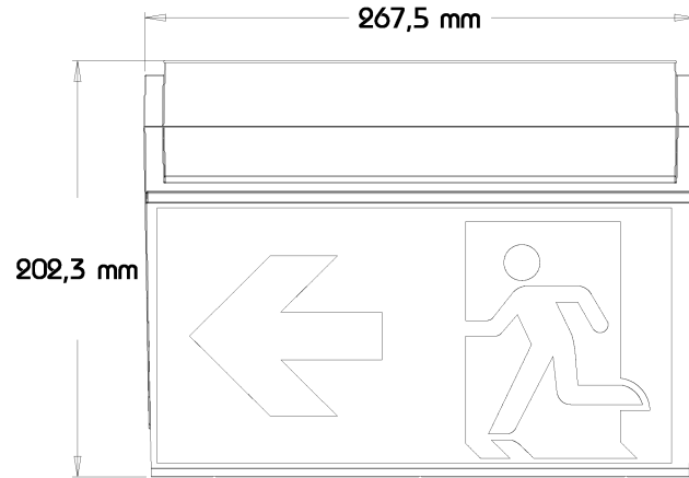
Ansicht Vorne
