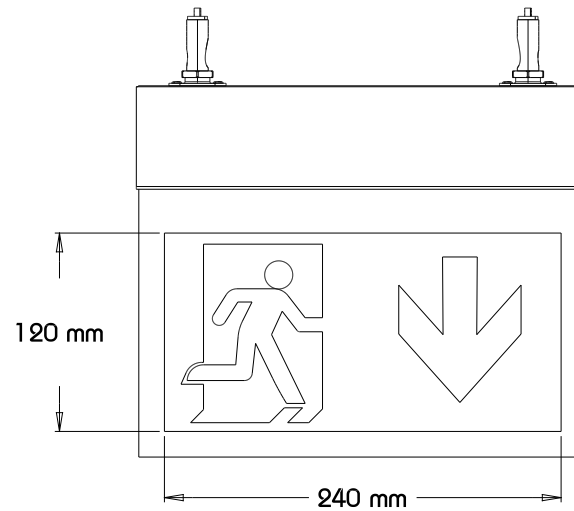
Ansicht Hinten
