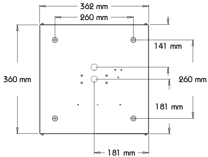
Ansicht Oben
