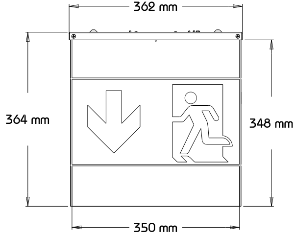
Ansicht Vorne
