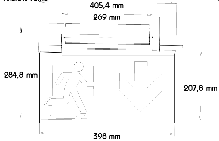
Ansicht Vorne
