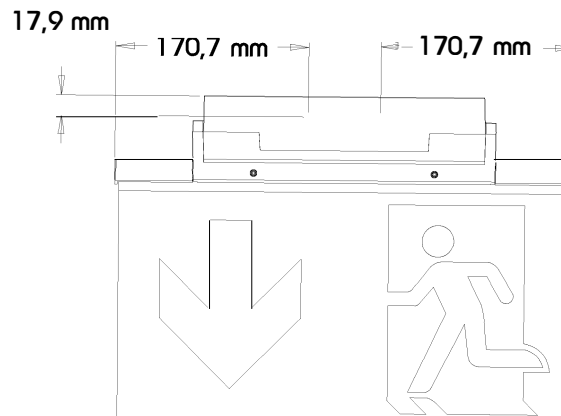
Ansicht Hinten
