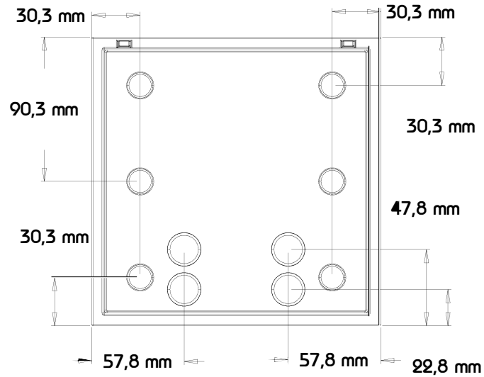
Ansicht Oben
