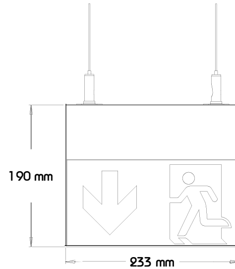
Ansicht Hinten
