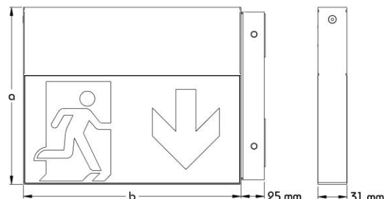
Maßzeichnung
